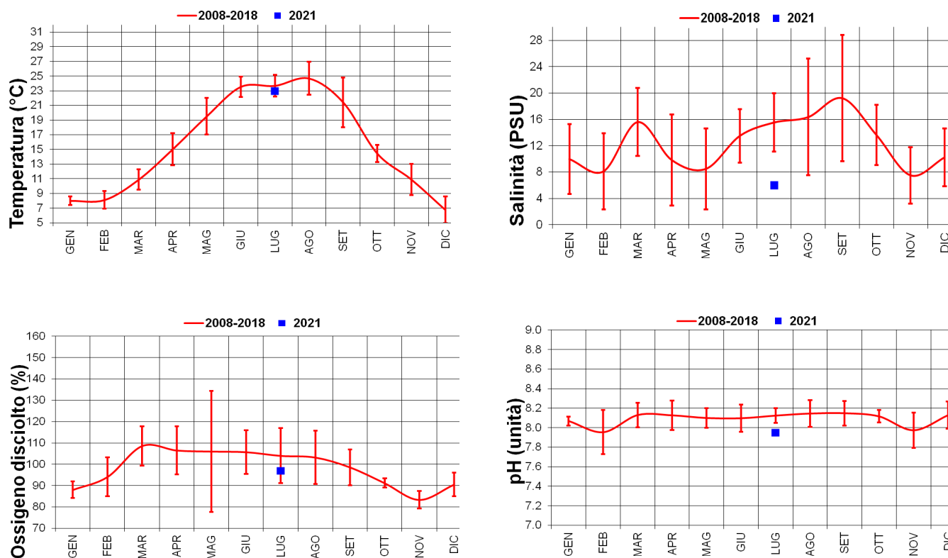
Figura 2 – Lagune di Caorle e Baseleghe. Confronto dell'andamento dei principali parametri chimico-fisici di luglio 2021 con la serie storica 2008 - 2018 (media ± dev.st.)
