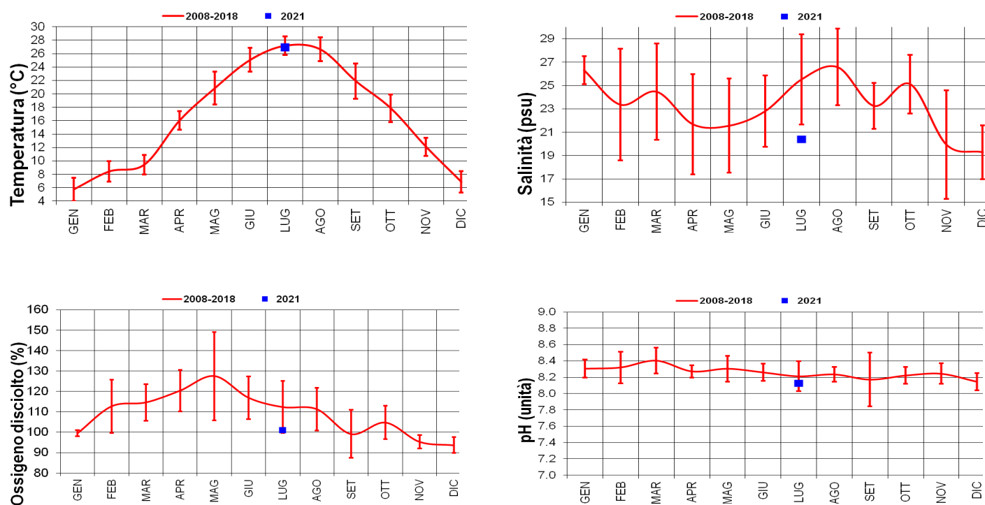
Figura 3 – Lagune del delta del Po. Confronto dell'andamento dei principali parametri chimico-fisici di luglio 2021 con la serie storica 2008-2018 (media \pm dev.st.)
